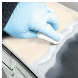
Aplikace utěrek BONDERITE M-NT 1455 W pouze na holý kov. Udržování vlhkého povrchu po dobu 2 min.
