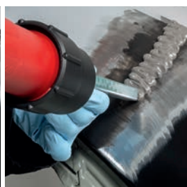
Nanesení produktu TEROSON EP 5010 TR
